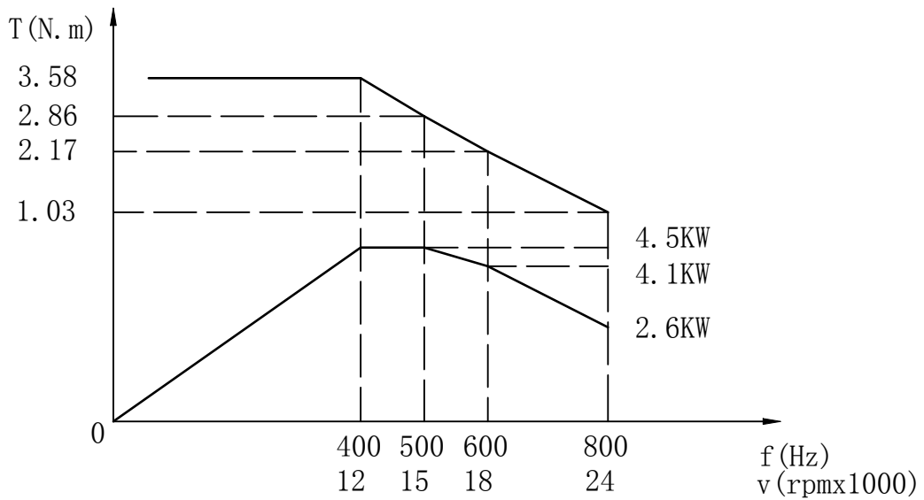
扭矩/功率曲线
