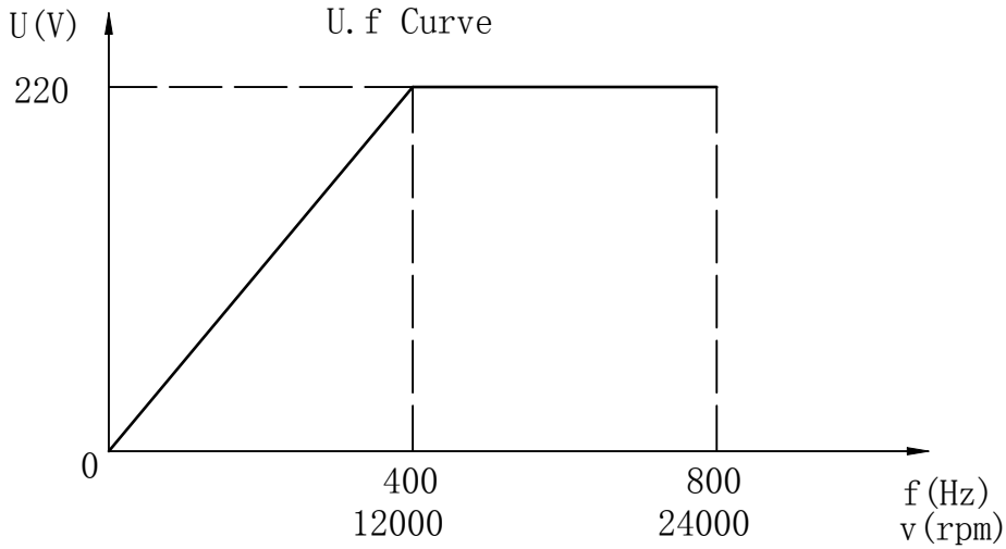
频压曲线
